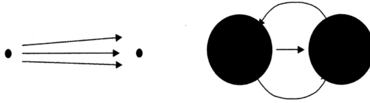
Рис. 6. Слева – локально однородное поле тяготения, справа – поле, которое нельзя считать однородным даже локально
