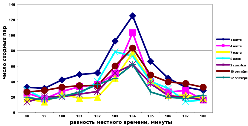
Рис. 7-8: Эффект синхронного по местному времени появления сходных гистограмм в Пушино и в на станции Новолазаревская в Антарктиде в разные дни от 1 марта до 22 сентября 2003 года. (Расчетная разность местного времени равна 104 минутам.)
