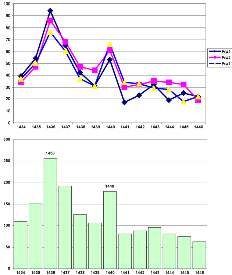
Рис. 22-11: Распределение числа пар сходных 1-минутных гистограмм в зависимости от величины разделяющего их интервала времени (минуты). Вероятность повторного появления гистограмм сходной формы изменяется с двумя различными суточными периодам — одним равным “солнечным суткам” (1440 минут) и другим, равным “звездным суткам” (1436 минут). Генераторы № 28 и № 37. Нижняя диаграмма — суммарное распределение. Верхняя — результаты трех отдельных сравнений. По оси абсцисс — интервалы времени между сходными гистограммами (минуты). По оси ординат — число сходных пар, соответствующее данной величине интервала.
