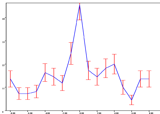
Рис. 3-17: Синхронность изменения формы 1-часовых гистограмм при измерении шумов в "Улитке" (ГАИШ, Москва) и при измерении альфа-активности ^{239}\text{Pu} в Пушкино 22 марта 2001 г. Указаны среднеквадратичные ошибки на основании оценки по Пуассону. Оси как на предыдущих рисунках.
