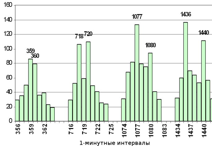
Рис. 13-3: Сравнение одномоментных гистограмм. При 4-х оборотах в сутки против часовой стрелки коллиматора, вырезающего узкий пучок альфа-частиц, вылетающих при радиоактивном распаде ^{239}\text{Pu} , сходные гистограммы реализуются с периодами соответствующими долям звездных и солнечных суток. Один оборот совершается за 360 минут. При этом вероятность реализации сходных 1-минутных гистограмм возрастает с периодом, равным 359 и 360 минутам. При совершении двух оборотов вероятность появления сходных гистограмм возрастает, соответственно, через 359 \times 2 = 718 минут и 360 \times 2 = 720 минут. При совершении трех оборотов эти величины равны 359 \times 3 = 1077 минутам и 360 \times 3 = 1080 минутам и при четырех оборотах равны 359 \times 4 = 1436 и 1440 минутам, соответственно. Измерения 27.05.2004–09.06.2004 г. Ордината — число сходных пар гистограмм; абсцисса — число 1-минутных интервалов.
