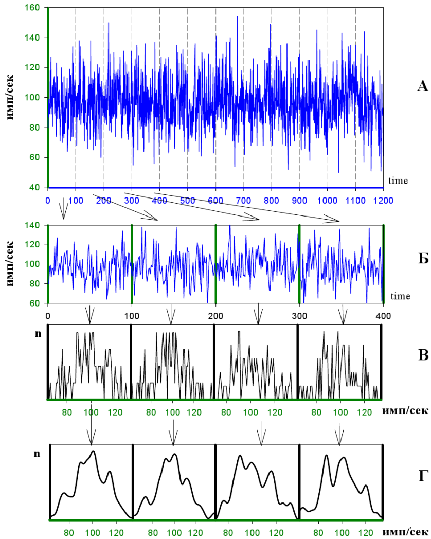
Рис. 2-4: А — изображен “растянутый” фрагмент временного ряда результатов измерения альфа-активности препарата ^{239}\text{Pu} . Б — временной ряд поделен на неперекрывающиеся отрезки по 100 последовательных чисел в каждом. В — для каждого отрезка построена гистограмма (оси абсцисс — величина активности имп/сек; по оси ординат число измерений, соответствующее данной величине активности). Г — закономерности проявляются в результате сглаживания “скользящим суммированием” или с “окном”, равным, например, 4.
