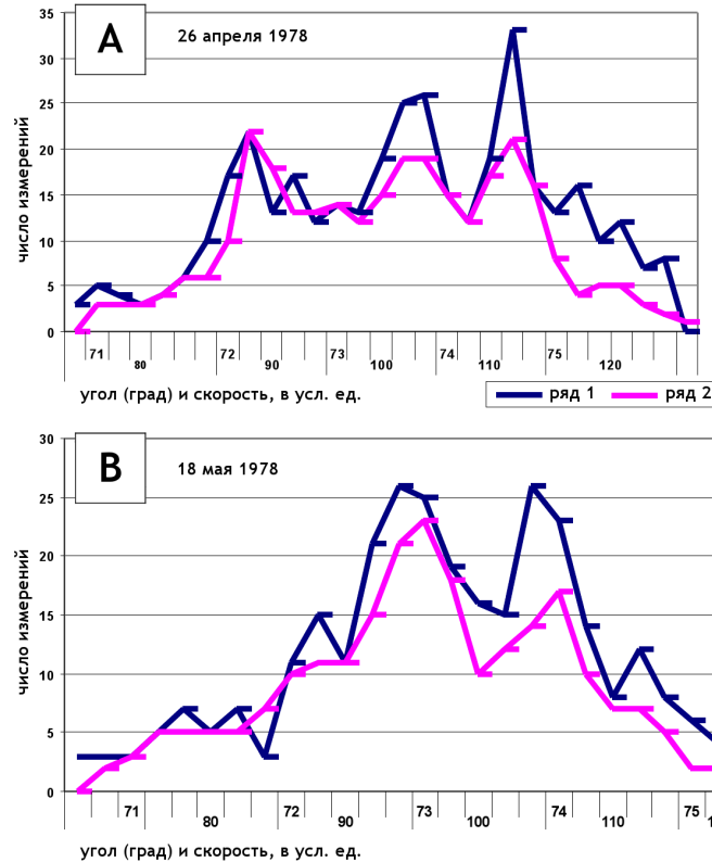
Рис. 20: Гистограммы, построенные по синхронным измерениям углов поворота лимба при настройке поляриметра (1) (В. Е. Жвирблис, Москва) и скорости крeатинкиназной реакции (2) в Пущино оказались сходными, как в опыте 26 апреля, так и в опыте 18 мая 1978 г. [92].
