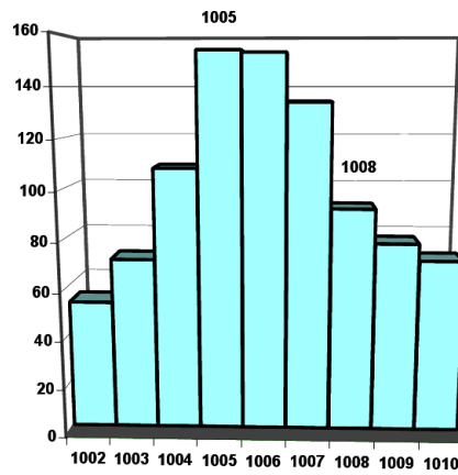
Рис. 16-11: В день зимнего солнцестояния 22 декабря 2000 г. сходные гистограммы появляются с периодом, равным продолжительности темного времени, скорректированным по соотношению длительности звездных и солнечных суток (1005, 1006 минут, а не 1008 минут).
