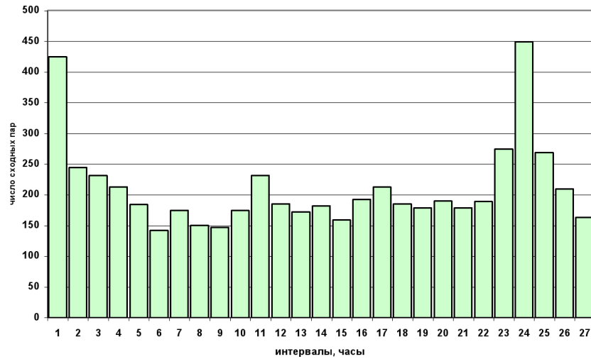
Рис. 5-1: Вероятность реализации 1-часовых гистограмм сходной формы в зависимости от интервала времени между ними. Измерения альфа-активности ^{239}\text{Pu} в марте-июле 2002 г. в Пуцино (таблица 5-1). По оси абсцисс — интервалы, часы. По оси ординат — число пар сходных гистограмм.
