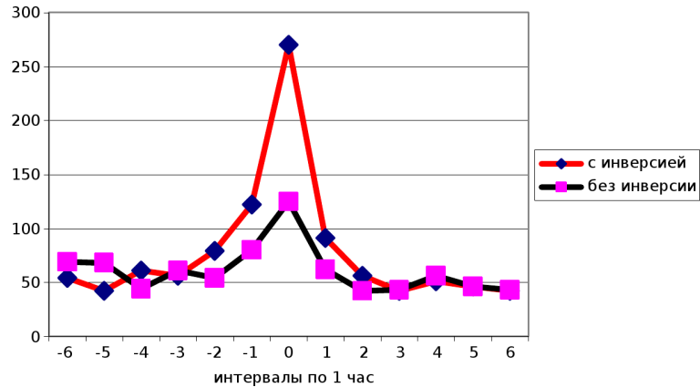
Рис. 20-8: Эффект палиндромов в эвекции. (Пояснения в тексте.)
