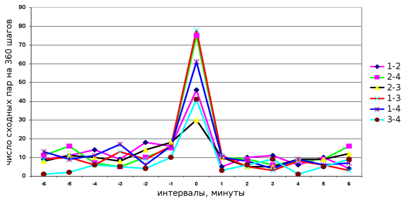
Рис. 7-15: В 1-минутных гистограммах (результаты измерений альфа-активности ^{239}\text{Pu} 15 октября 2005 г. в Пуцшино счетчиком с коллиматором, направленным на Полярную звезду, и в Новолазаревской счетчиком без коллиматора) наблюдается: 1) “сильная” абсолютная синхронность изменения гистограмм при измерениях в Пуцшино (№ 1): при измерениях без коллиматора и в Пуцшино с Западным коллиматором (№ 3); 2) “сильная” абсолютная синхронность в Пуцшино с коллиматором, направленным на Солнце (№ 2) и в Новолазаревской (без коллиматора) (№ 4); 3) “средняя” абсолютная синхронность при измерениях в Пуцшино (№ 1) и в Новолазаревской (№ 4) без коллиматоров; 4) “слабая” абсолютная синхронность при измерениях в Пуцшино с Западным коллиматором (№ 3) и в Новолазаревской без коллиматора (№ 4); 5) “слабая” абсолютная синхронность в Пуцшино без коллиматора (№ 1) и счетчика с Солнечным коллиматором (№ 2). 6) № 2–3: отсутствует абсолютная синхронность при измерениях в Пуцшино с “солнечным” (№ 2) и “Западным” (№ 3) коллиматорами, находящимися рядом в Пуцшино.
