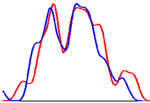
Рис. 18-3-17: Полнолуния 27 апреля и 25 июня 2002 года за 2 минуты до моментов максимума.
