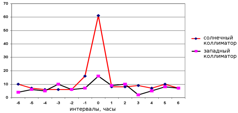
Рис. 7-14: При построении 60-минутных гистограмм по результатам измерений альфа-активности ^{239}\text{Pu} в Пуцшино счетчиком с коллиматором, направленным на Солнце, и в Новолазаревской счетчиком без коллиматора (также как при построении 1-минутных гистограмм) наблюдается четкая абсолютная синхронность с Антарктикой. При измерениях в Пуцшино счетчиком с коллиматором, направленным на Запад совсем нет абсолютной синхронности.
