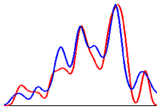
Рис. 18-3-5: Полнолуния 27 февраля и 23 августа 2002 года в моменты максимума. “Явное” сходство, но снова зеркальный поворот.
