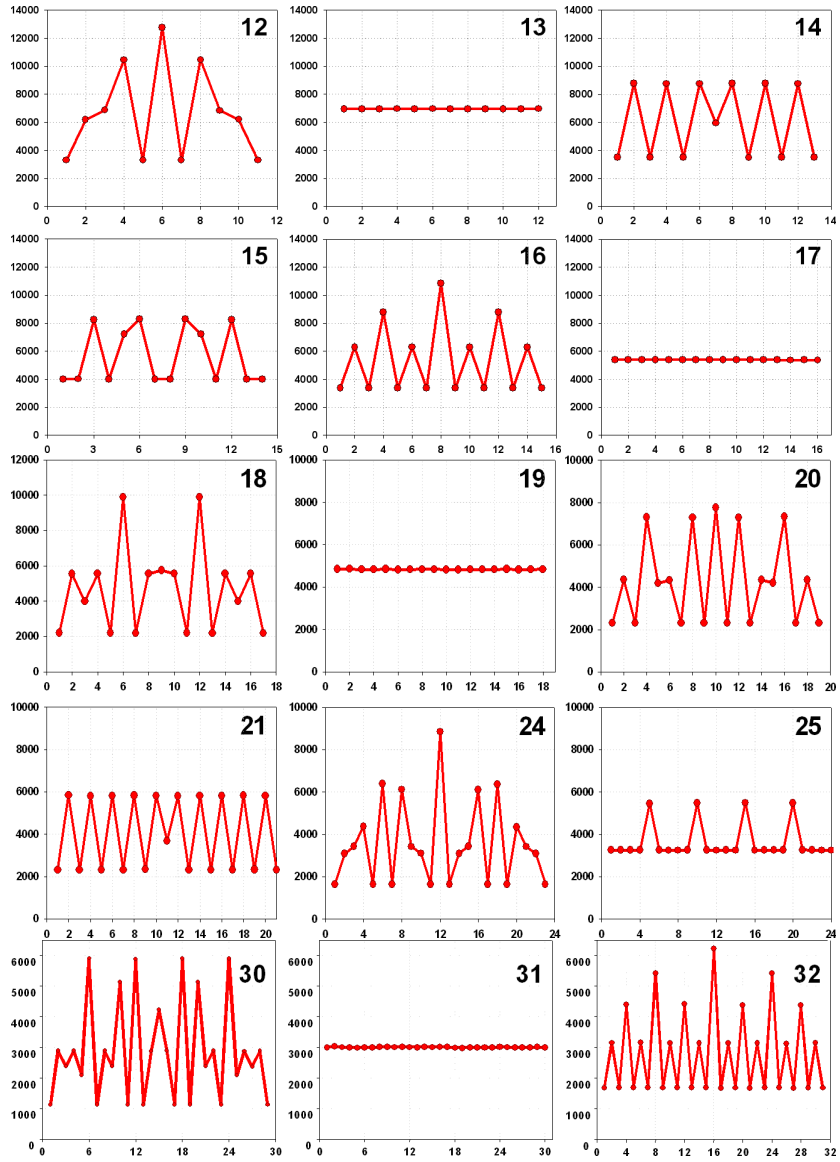
Рис. 24-2: Распределение числа сомножителей внутри разрядов, соответствующих разным системам счисления. Числа в верхних углах рисунков — величины отрезков натурального ряда сомножителей.
