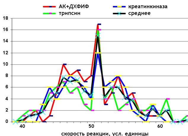
Рис. 8: Иллюстрация сходства формы гистограмм в опытах с АК + ДХФИФ (18 января 1979 г.), трипсином (31 января 1979 г.) и креатинкиназой (26 декабря 1978 г.). Гистограммы сходной “идеи формы” наблюдаются при измерениях скоростей ферментативных реакций катализируемых трипсином или креатинкиназой и реакции аскорбиновой кислоты (АК) с дихлорфенолиндофенолом (ДХФИФ).
