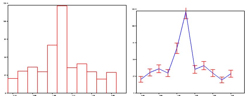
Рис. 15-6: При выравнивании временных рядов по “лунному восходному времени” — по времени восхода Луны, выявляется корреляция формы гистограмм с положением Луны относительно горизонта.
