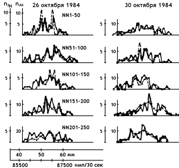
Рис. 36: Опыты 26 и 30 октября 1984 г. Синхронные по местному времени измерения бета-активности {}^3\text{H} в Ленинграде ( 59^\circ 57' с.ш. и 30^\circ 12' в.д., А. Ю. Сунгуров) и скорости реакции АК + ДХФИФ в Пущино (С. Э. Шноль, Н. П. Иванова и Т. Я. Брицина), рис. 25 из [32, 33].
