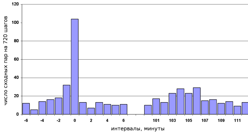
Рис. 7-11: При построении 1-минутных гистограмм по результатам измерений альфа-активности ^{239}\text{Pu} в Пущино счетчиком с коллиматором, направленным на Солнце и без коллиматора в Новолазаревской наблюдается синхронность по абсолютному времени и отсутствует абсолютная синхронность Измерения 24 января 2008 г.
