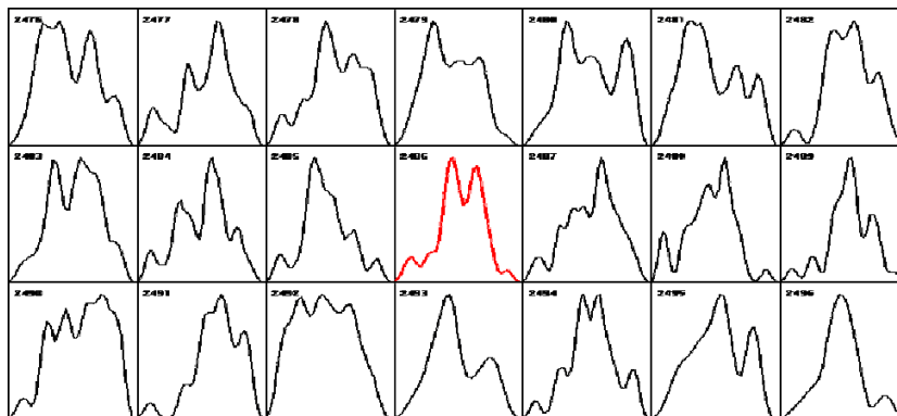
Рис. 22-16: Ряд 0,5-минутных гистограмм, построенных по результатам измерений 8 апреля 2005 г. генератором GCP № 103 (Рик Бергер, Сан Антонио, Техас, США, 29,493° с.ш. и 98.6127° в.д.) Расчетный момент максимума затмения № 2486, гистограмма характерной формы реализуется точно в этот момент.
