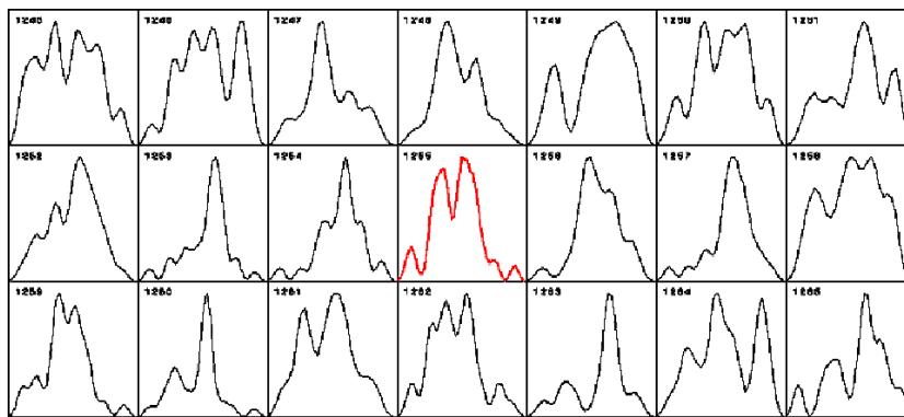
Рис. 22-17: Ряд 0,5-минутных гистограмм, построенных по результатам измерений 3 октября 2005 г. генератором GCP № 28 (Роджер Нельсон, Принстон, Нью Джерси, США, 40°35' с.ш. и 74°65' з.д.). Расчетный момент максимума затмения № 1256, гистограмма характерной формы реализуется на 0,5 минуты позже (1255).
