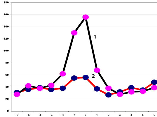
Рис. 21-10: При вращении коллиматора, совершающего вместе с Землей 4 оборота в сутки против часовой стрелки, “искусственные сутки” равны 6 часам. Мощный эффект полусуточного палиндroma наблюдается при сравнении рядов “дневных” 3-х часовых гистограмм с рядами инвертированных (1) и не наблюдается при сравнении с рядами неинвертированных (2) 3-х часовыми “ночными” гистограмм. Сумма двух опытов 29–30 и 30–31 мая 2004 г.
