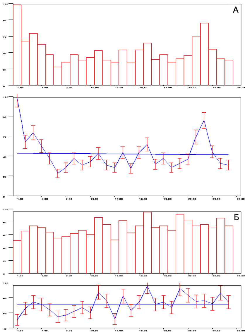
Рис. 11-1: При измерениях в Пушино ( 54^\circ с.ш.) альфа-активности препаратов ^{239}\text{Pu} прибором с коллиматором, вырезающим поток альфа-частиц, вылетающих при радиоактивном распаде в направлении на Полярную звезду ( 90^\circ с.ш.), исчезает эффект ближней зоны и околосуточный период изменения формы 60-минутных гистограмм.
