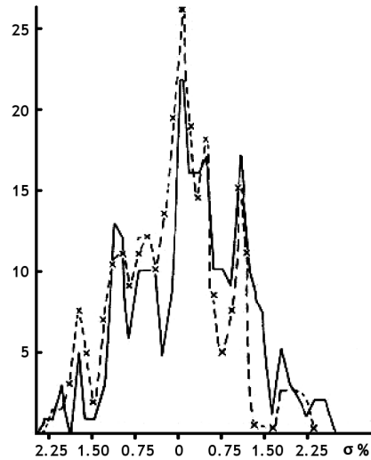
Рис. 32: Форма гистограмм не зависит от природы измеряемого процесса. Измерения бета-активности ^{14}\text{C} (В. И. Брусов) и скорости реакции АК + ДХФИФ (С. Э. Шноль, Т. Я. Брицина и Н. П. Иванова). Опыт 4 июля 1984 г. Ось абсцисс для обоих процессов — в долях среднеквадратичного отклонения ( \sigma ), рис. 19 из [32].
